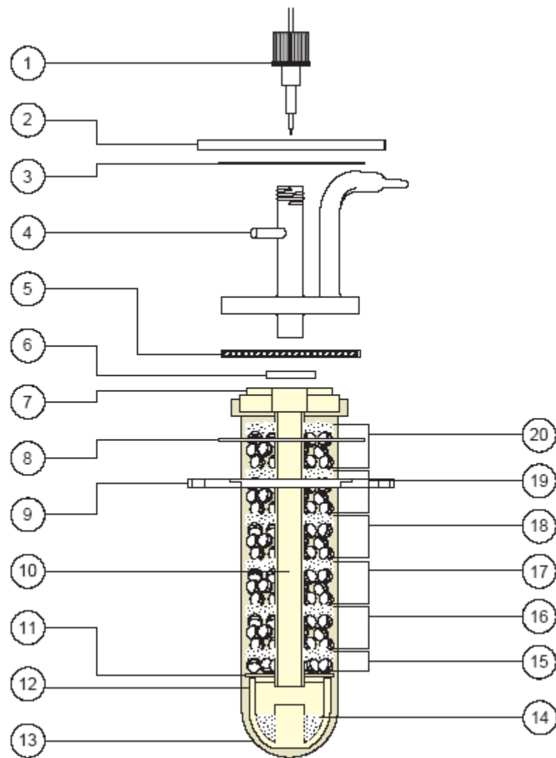
图 2-27 组装反应器
